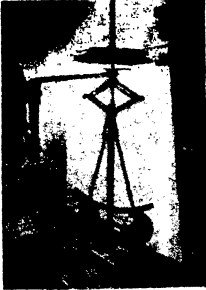
جهاز التحكم الآلي في سرعة الآلة البخارية الذي اخترعه جيمس وات .
